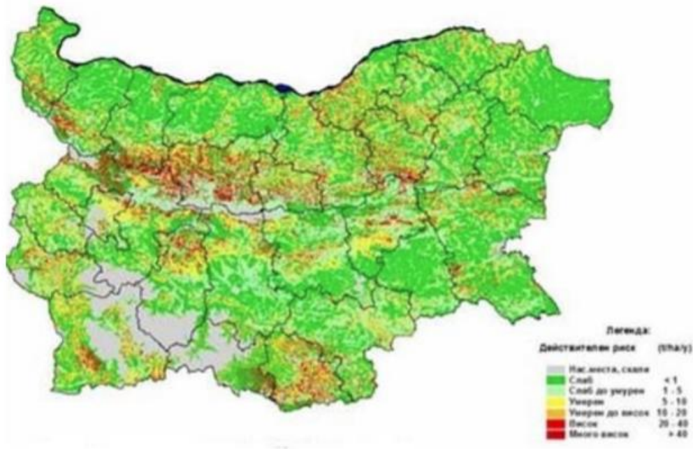
Фигура 3 Водоплощна ерозия в България
