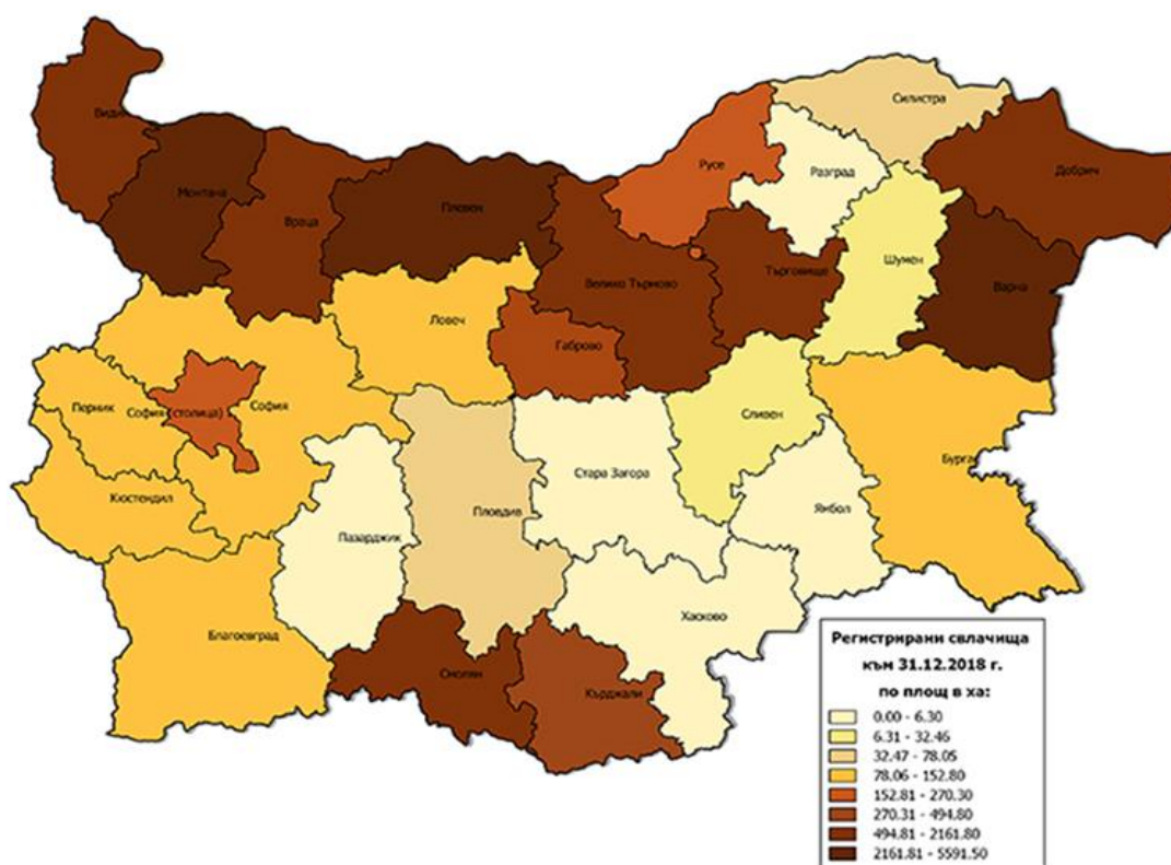
Фигура 10 Разпределение на площите засегнати от свлачищни процеси в България, ха
