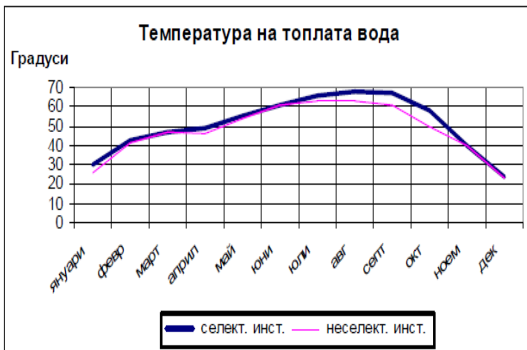
Фигура 15: Температура на произведената топла вода по месеци от селективна и неселективна инсталация
