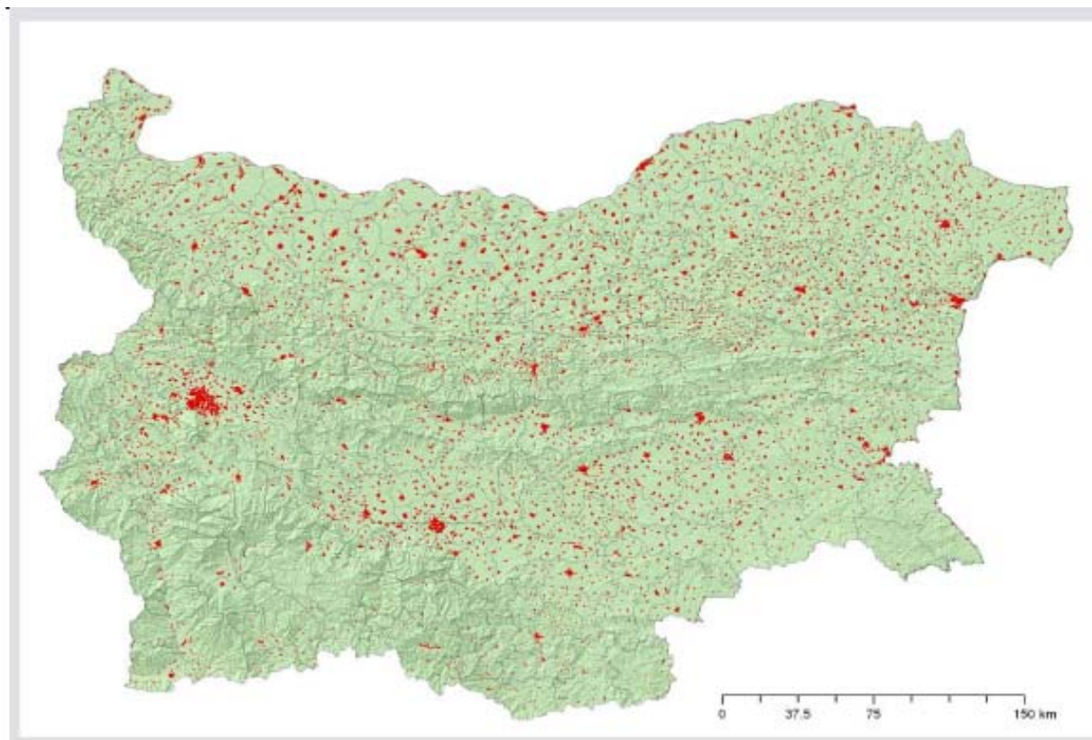
Фигура 20. Подходящи места за оползотворяване потенциала на слънчевата радиация за производство на енергия, отчитайки всички поставени ограничения
