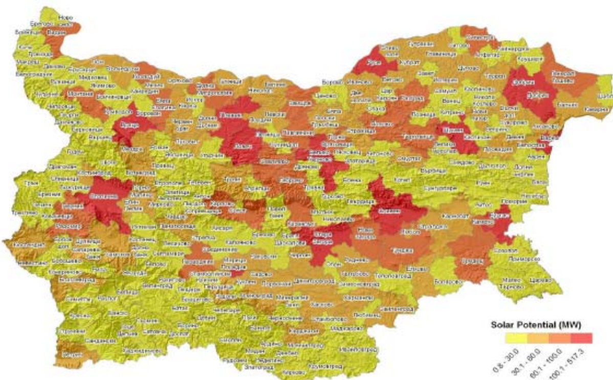
Фигура 19. Потенциал на слънчевата радиация в MW на общинско ниво
