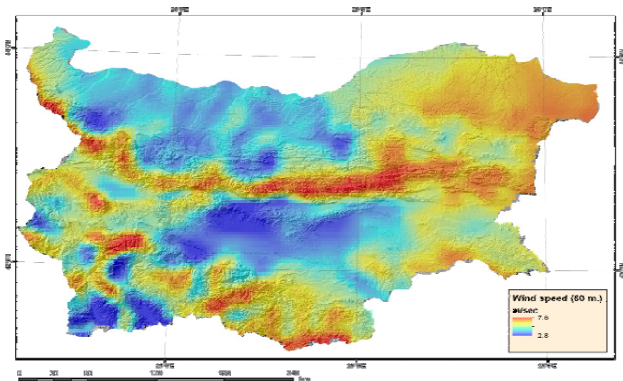
Фигура 10. Скорост на вятъра на височина 80 м
